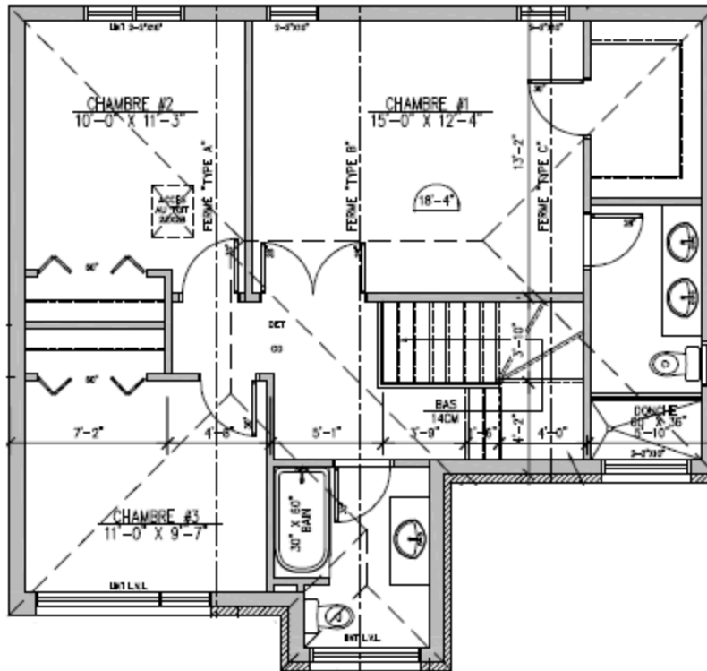
ÉTAGE : +/- 813 P.C.
