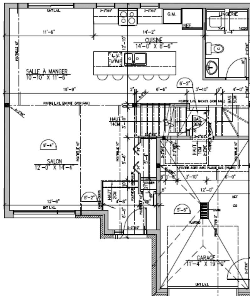
R-D-C : +/- 758 P.C.
